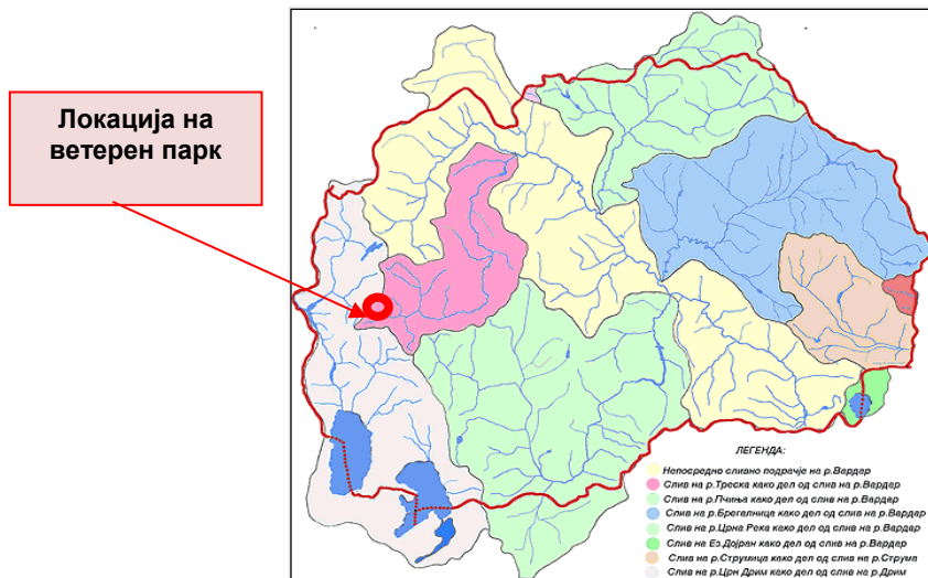
Слика 24 Хидролошка карта на Република Македонија
