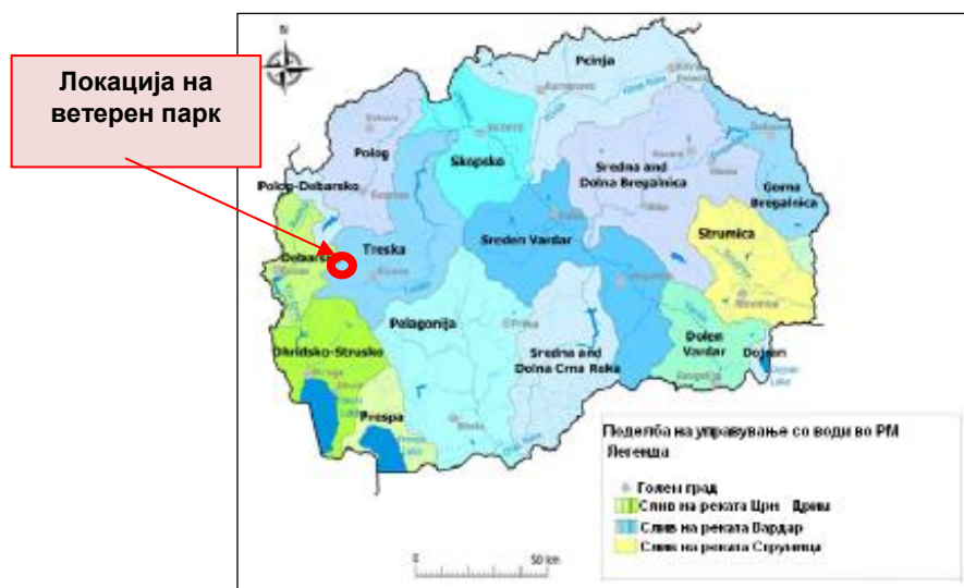
Слика 25 Водостопански подрачја во РМ
